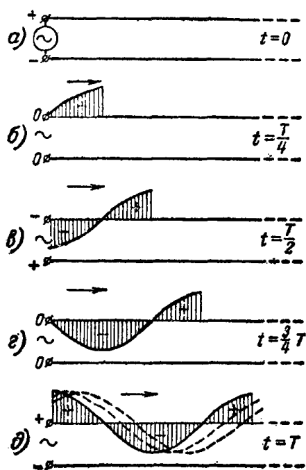
图 2.3 传输线中的行波
