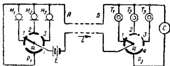
圖 1. 通路時間划分的多路电话
