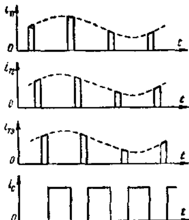
圖 3. 在受話器和同步設備中的电流
