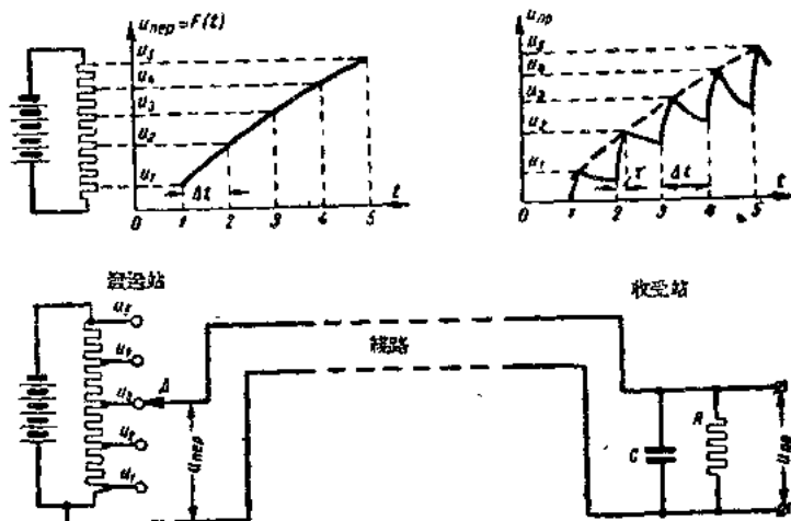
图 5. 用一系列离散值傳送电位器滑触子上的电压变化
