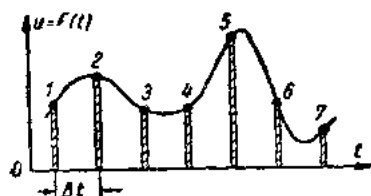
图 4. 用一系列离散值傳送信号
