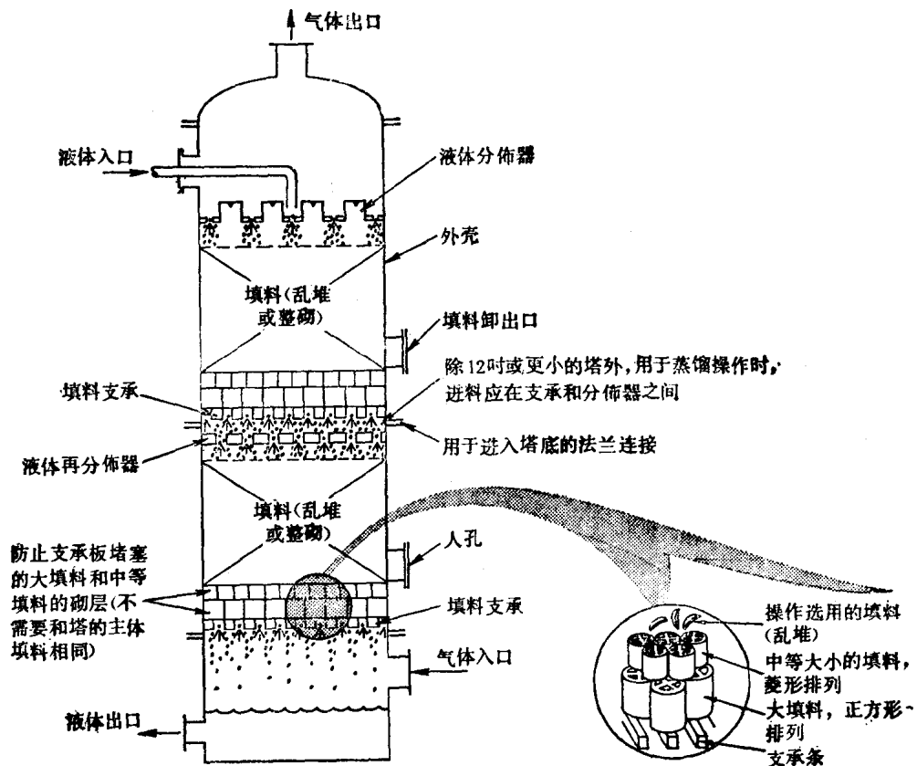
图 2-1(a) 填料塔结构示意图
