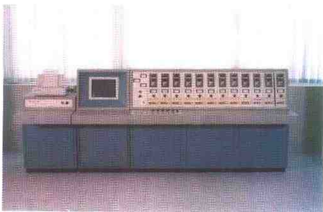
玻璃配料微机控制系统
