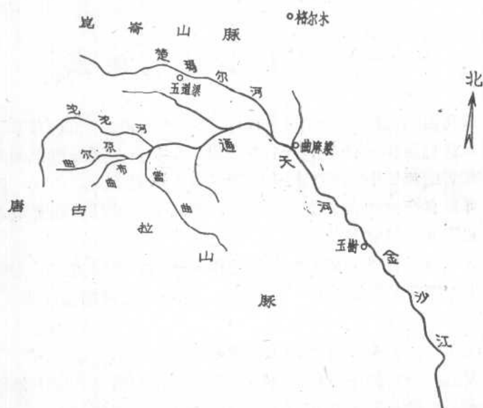
图1-1 长江河源图
