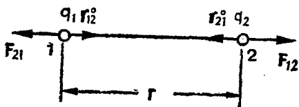
图 1.1 库仑力
