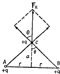
图 1.3 两点电荷垂线上的场强
