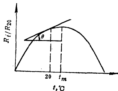
图 13-2-4 电阻随温度变化的抛物线特性
