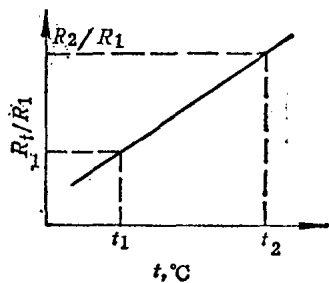
图 13-2-3 电阻随温度变化的直线特性
