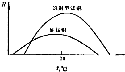
图13-2-1 通用型锰铜和硅锰铜的电阻对温度的关系
