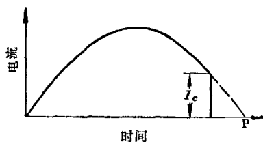
图 13.1-1 截止电流示意图
