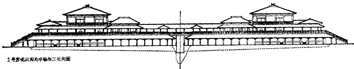
第一遗址整体复原南立面图
