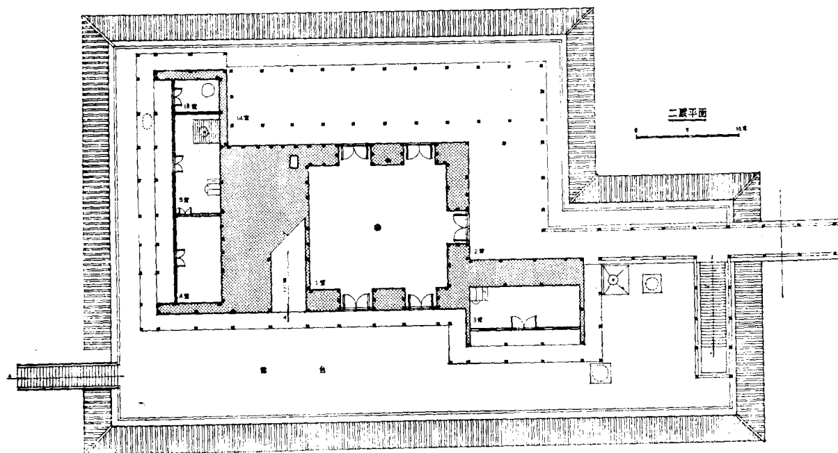
第一号宫殿遗址上层复原平面图
