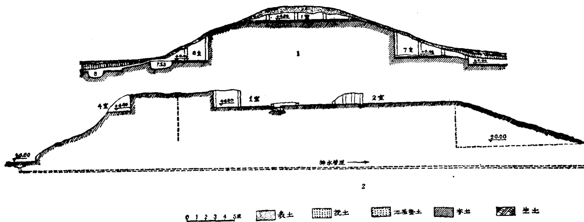
一号建筑遗址纵(2)横(1)剖面图
