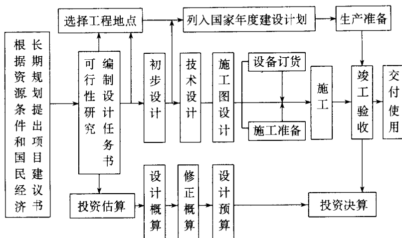
图 1.1 我国现阶段建设项目程序
