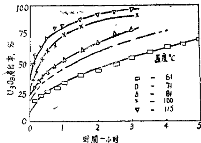
圖 3 用 5% \text{Na}_2\text{CO}_3 溶液及 2 公斤/厘米 2 氧壓下浸出 瀝青鈾礦時溫度對浸出速率的影響
