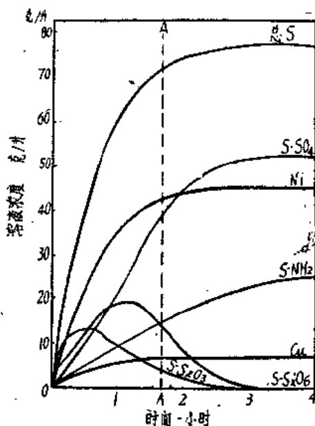
图 5 在氧压下用氨的水溶液浸出硫化 Cu-Ni-Co 精矿。 浸出时铜、镍及硫的化合物浓度的变化
