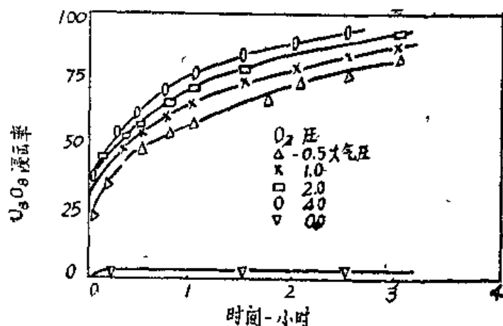
圖 2 用 5% \text{Na}_2\text{CO}_3 及 100^\circ\text{C} 溶液浸出瀝青鈾礦時 氧分壓對浸出速率的影響
