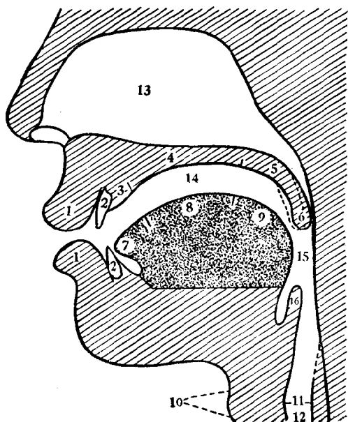
发音器官图
