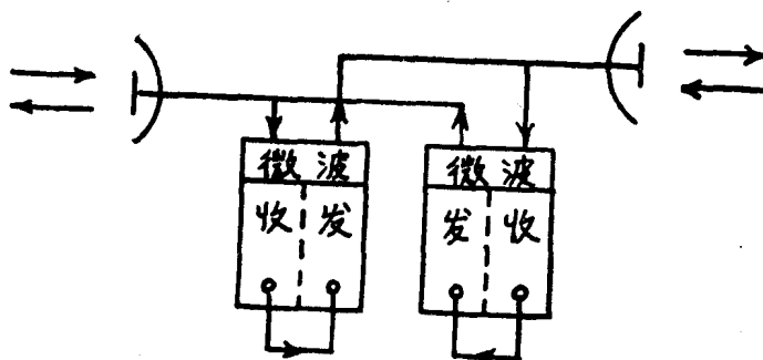
图 1-7 中继站示意图
