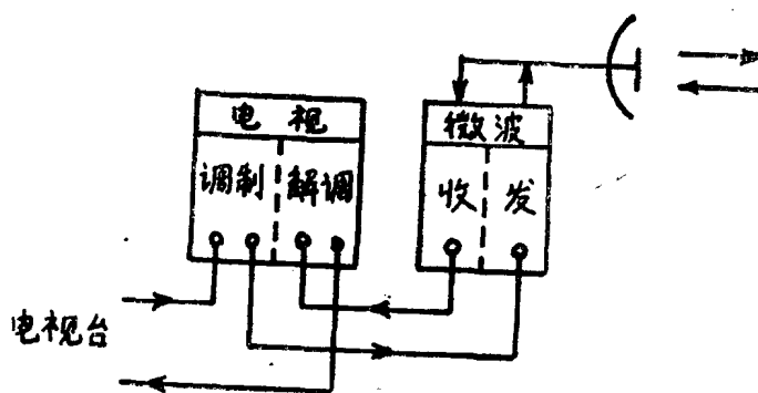
图 1-6 端站示意图
