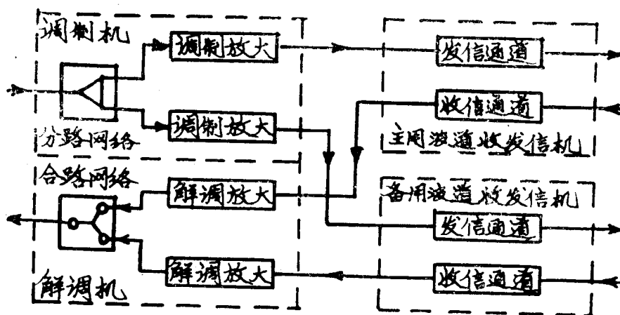
图 1-8 8 GHz 波道备用方框图
