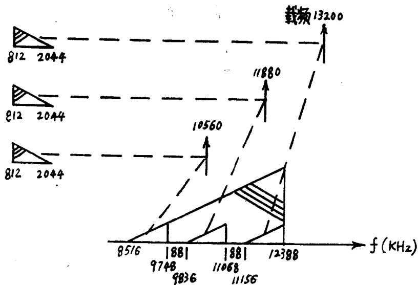
图 1-5 超主群标准频谱的构成
