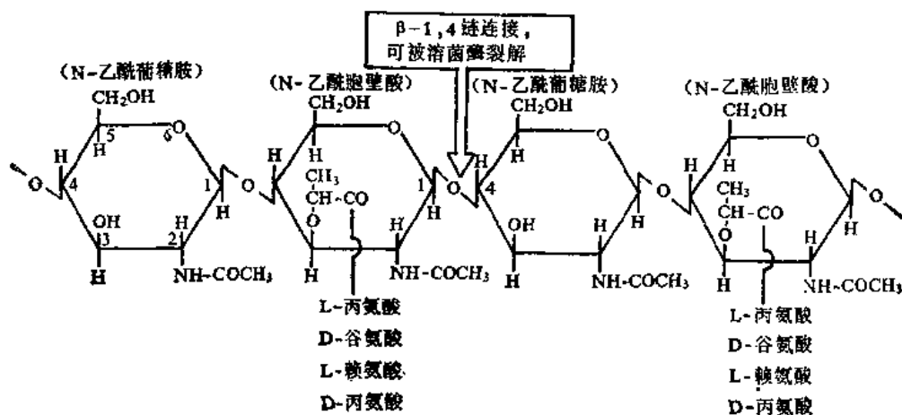
图 1-3 肽聚糖的结构
