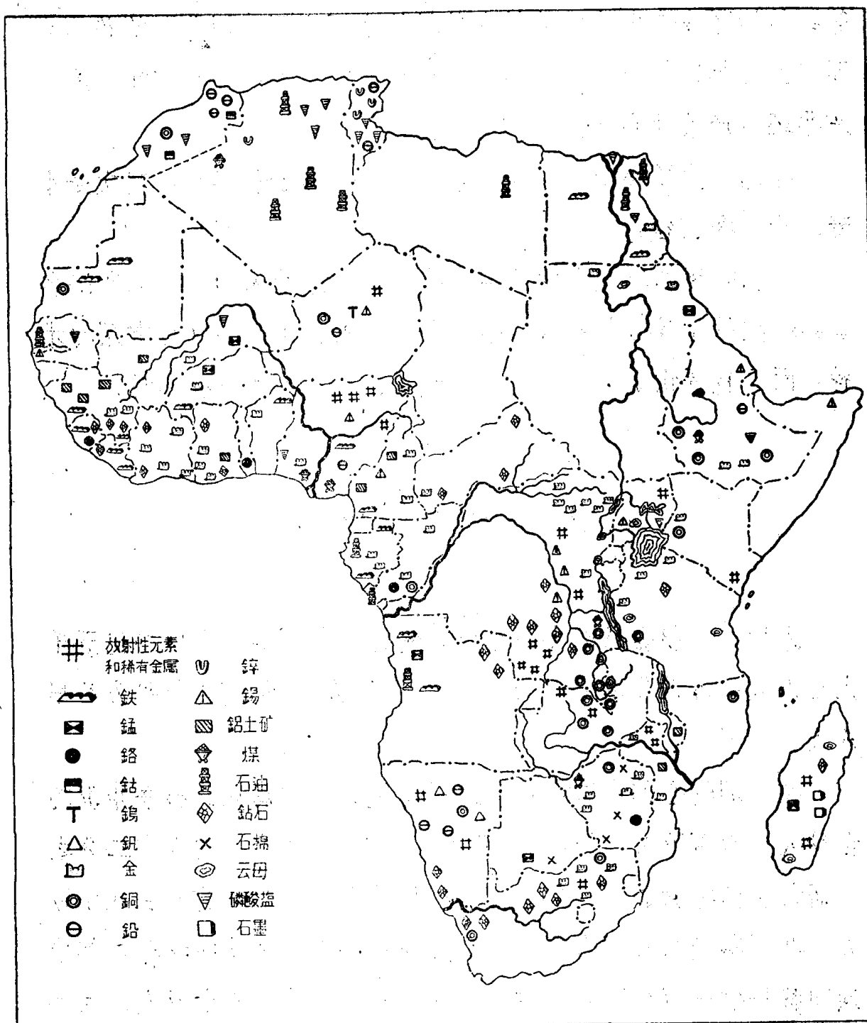
〔图四〕 非洲矿产分布图
