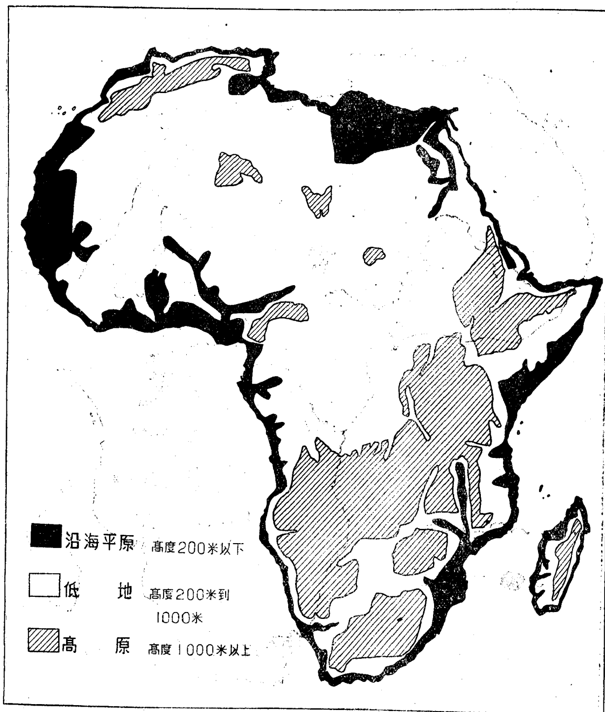
〔图一〕 非洲地形示意图
