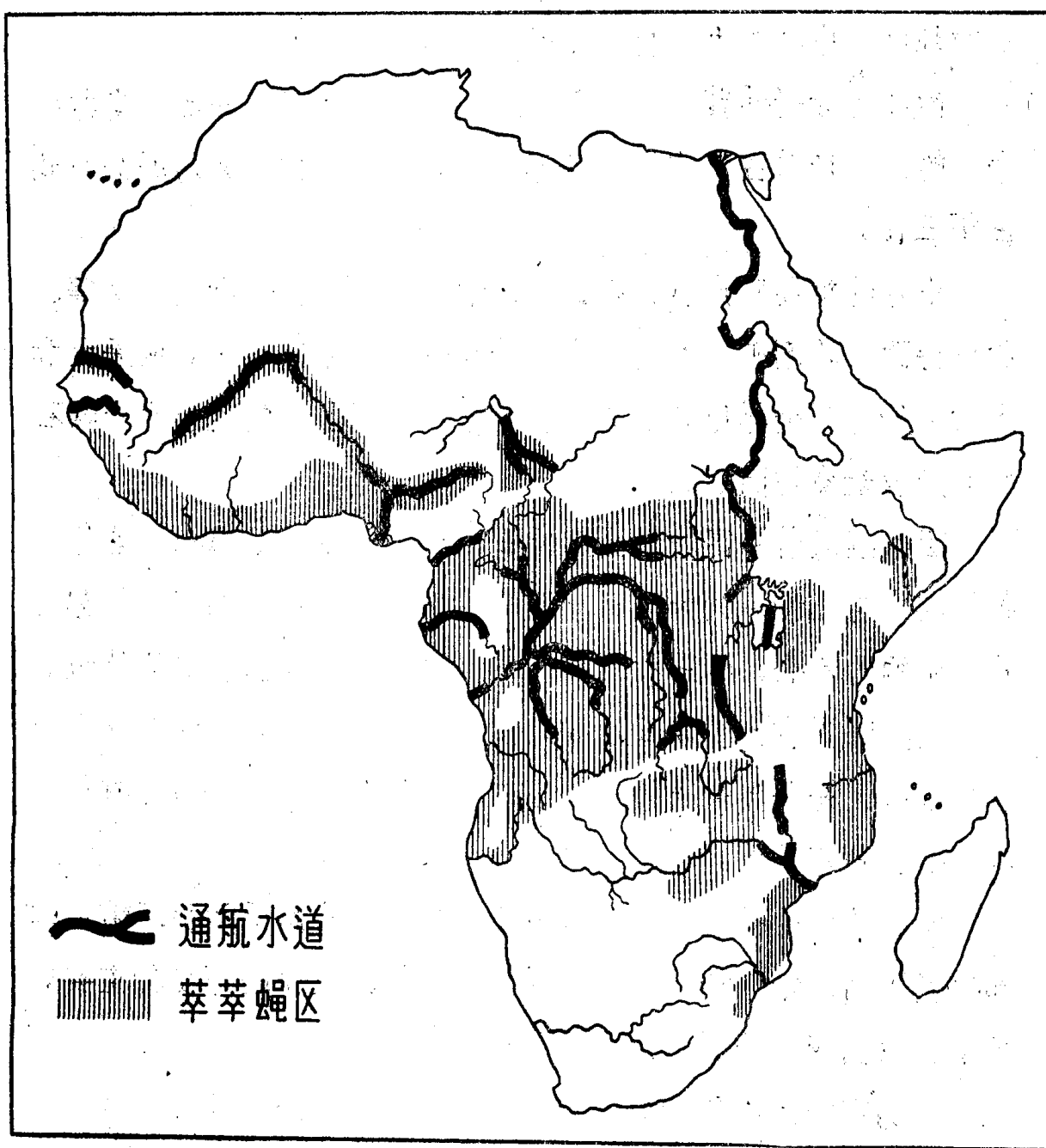
〔图三〕 非洲萃萃蝇繁殖区示意图
