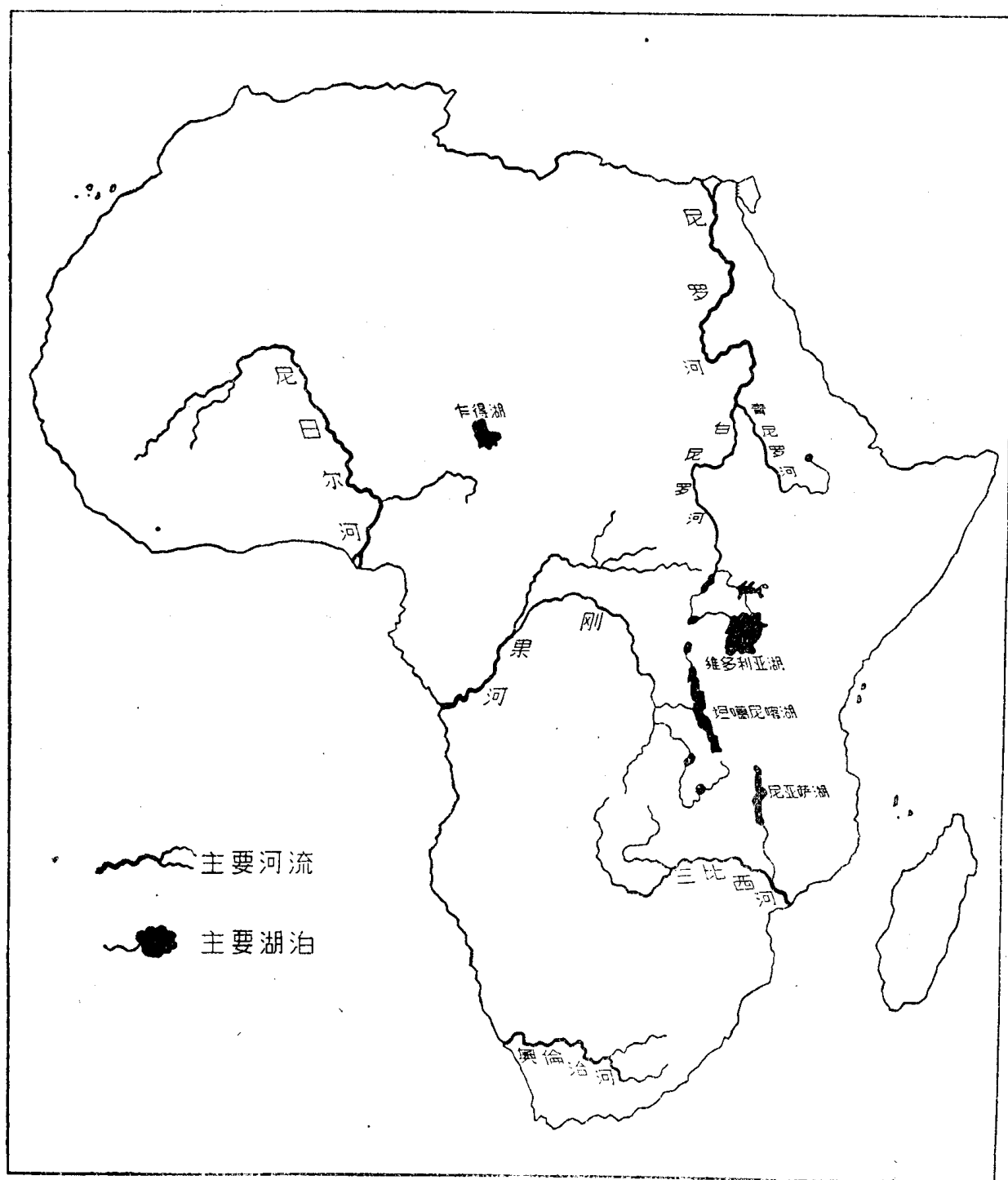
〔图二〕 非洲河流、湖泊分布图
