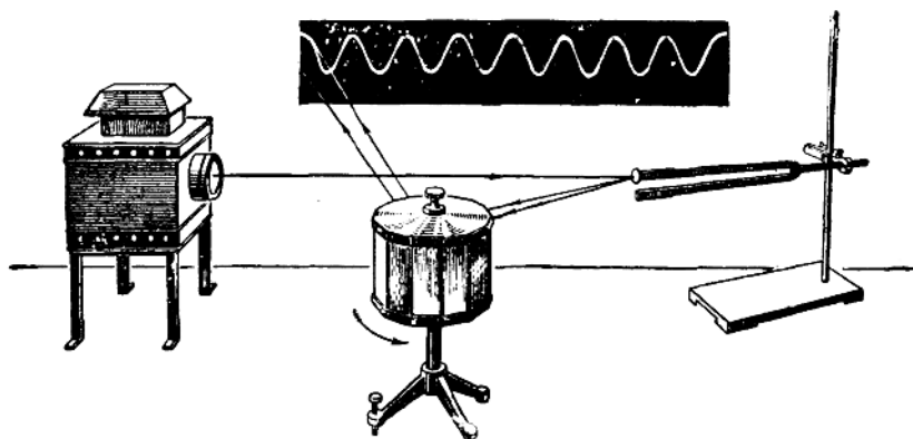
圖 4. 與圖 3 同，但加上水平掃射。
