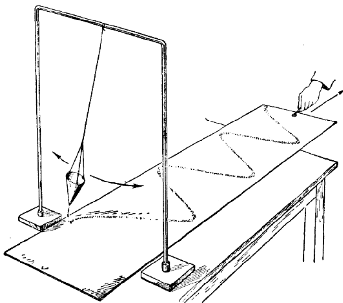
圖 1. 自錄擺。
