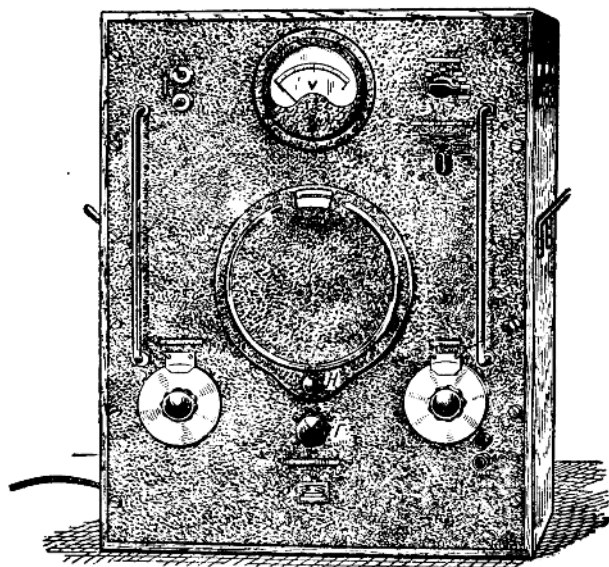
圖 9. 聲頻振盪器。
