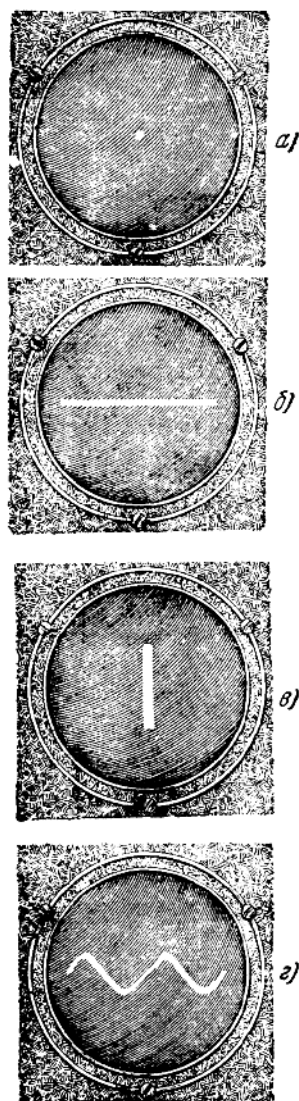
圖 7. 示波器螢光幕上的圖形:a—接上電子管, b—接上掃退電路, c—接上市電電源, d—接上掃退電路和市電電源。
