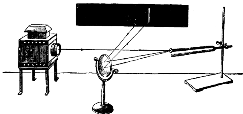
圖 3. 音叉發聲時光映的垂直掃射。
