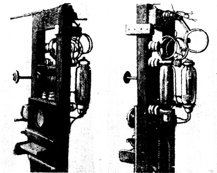
圖 11. 示範用高頻振盪器: a —控制板一邊的外貌, б —振盪迴路一邊的外貌。
