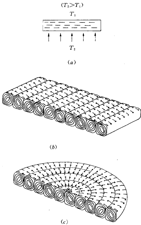
图 1.1 Bénard 流实验的示意图
