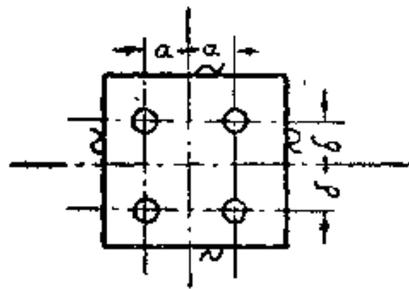
圖 20 利用螺絲孔定中心線
