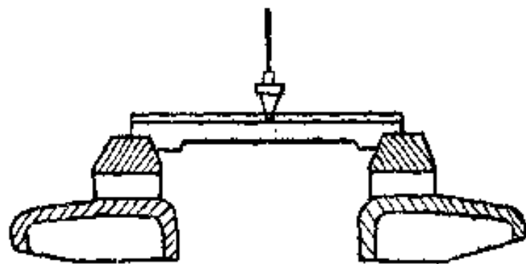
圖 19 利用樣板根據二底座之共同中心標點來找正底座的位置
