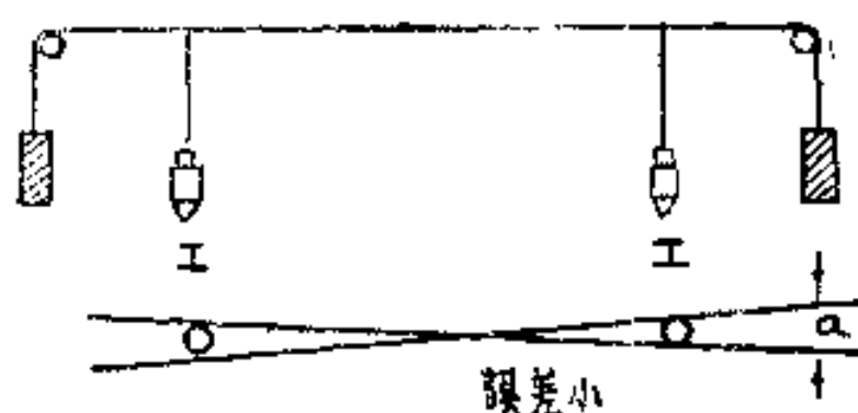
圖 10 用掛線法找平
