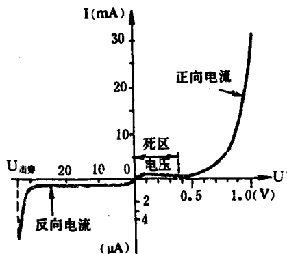
图 2-1 半导体二极管的伏安特性
