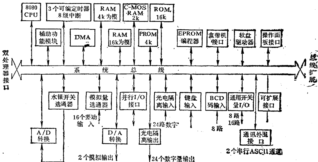
图1-1 SAM系统框图
