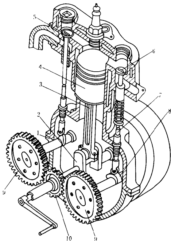
图 0-1 单缸内燃机
