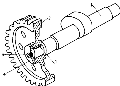
图 0-3 齿轮-凸轮轴
