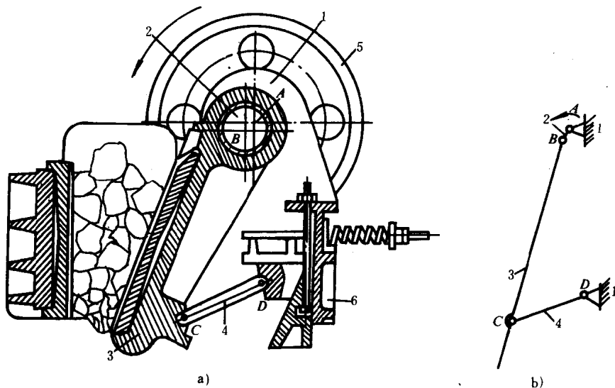
图 1-5 颚式破碎机及其机构运动简图
