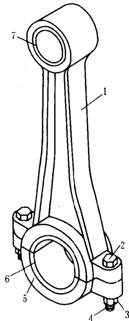
图 0-2 内燃机连杆
