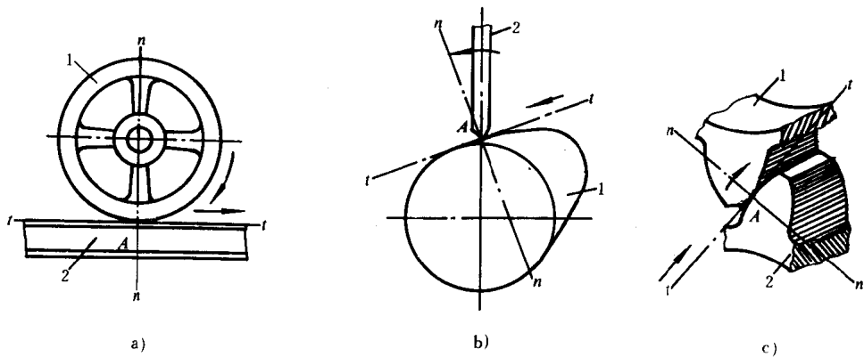
图 1-4 平面高副
