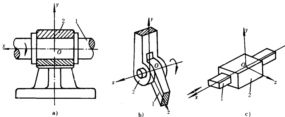
图 1-3 平面低副
