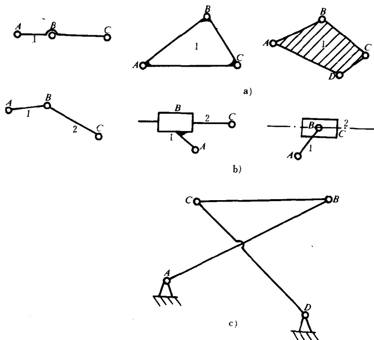
图 1-6 机构简图符号示例
