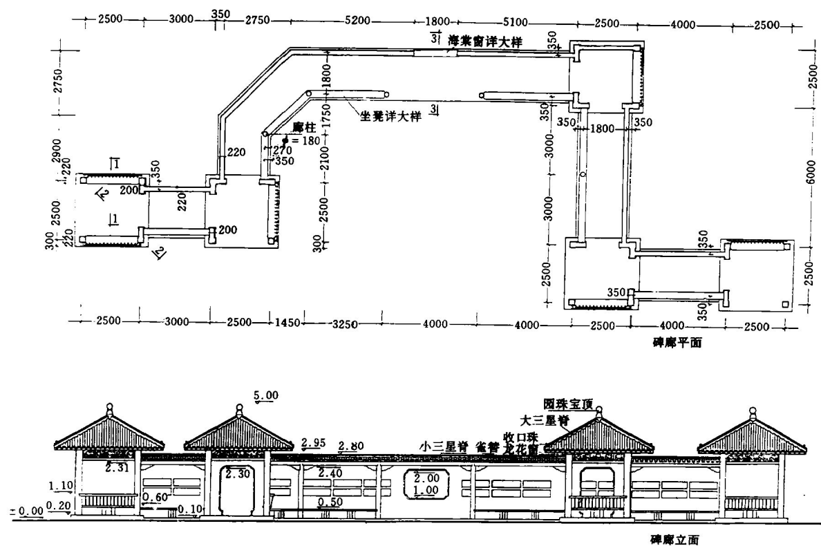
图 13 碑廊平、立面图
