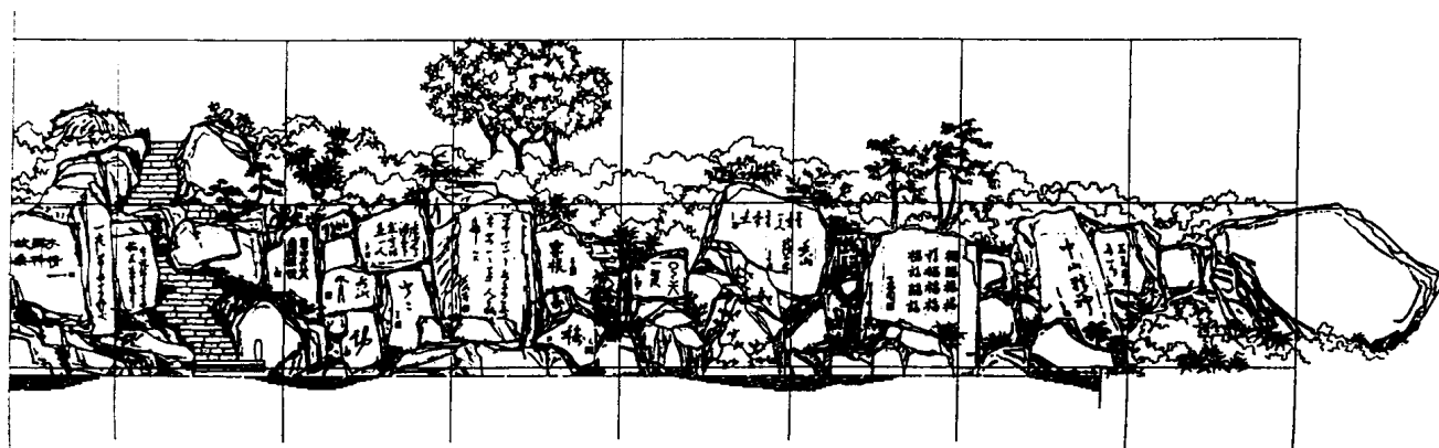
图 12 摩崖石壁西立面之二
