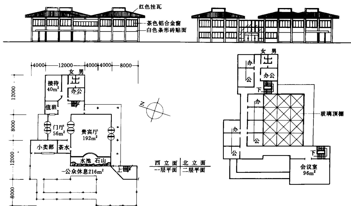
图 3 名木园综合楼平、立面图
