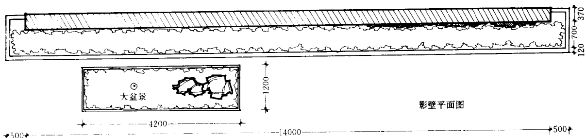
图 20 影壁平面图
