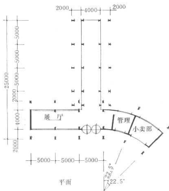
图7 翠苑入口门廊平、立面图
