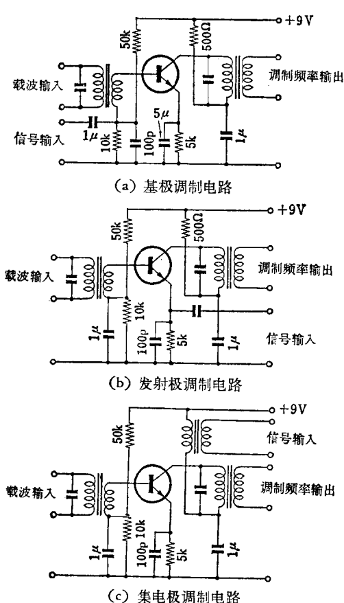
图 10-1 用三极管做的载波输出的双边带调制器
