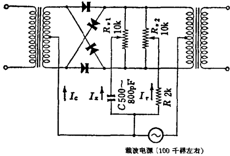
图 10·13 利用补偿电流法抑制载波漏泄的电路
