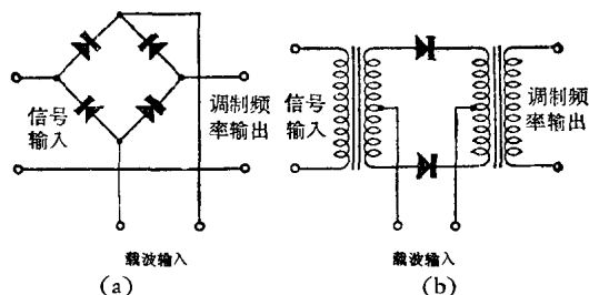
图 10-6 并联调制器
