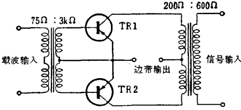
图 10·12 利用开关作用的晶体三极管调制器
