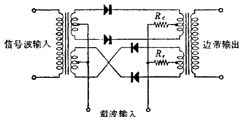
图 10·10 双平衡调制器
