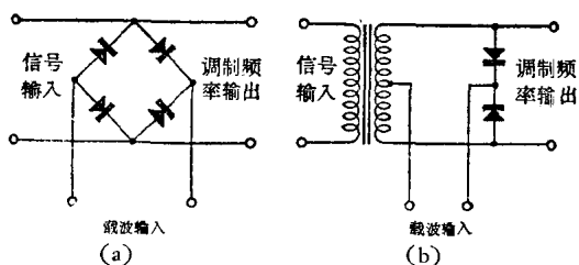
图 10-5 串联调制器
