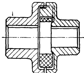
水泵用爪形弹性联轴节
