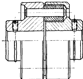
简单型弹性圈柱销联轴节
