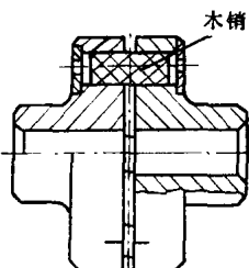
木销联轴节
