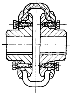
轮 胎 联 轴 节
