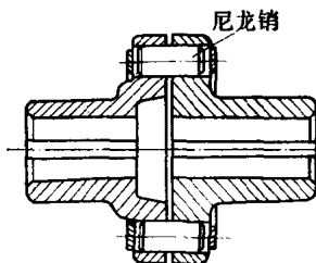
尼龙柱销联轴节
