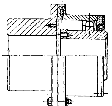
CLZ 型
