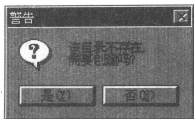
图 1.8 警告对话框
