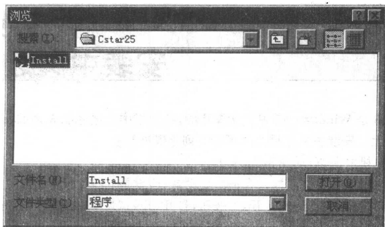
图 1.3 “浏览”对话框
