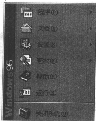
图 1.1 “开始”菜单
