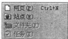
图 2.8 “新建”菜单
