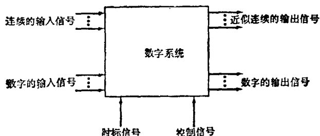
图 1-0 数字系统的一般形式
