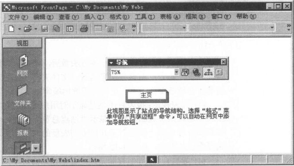
图 1-13 导航视图
