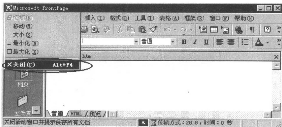
图 1-3 控制菜单
