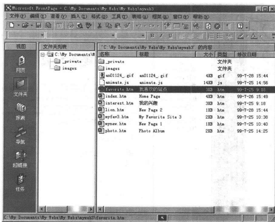
图 1-2 文件夹视图
