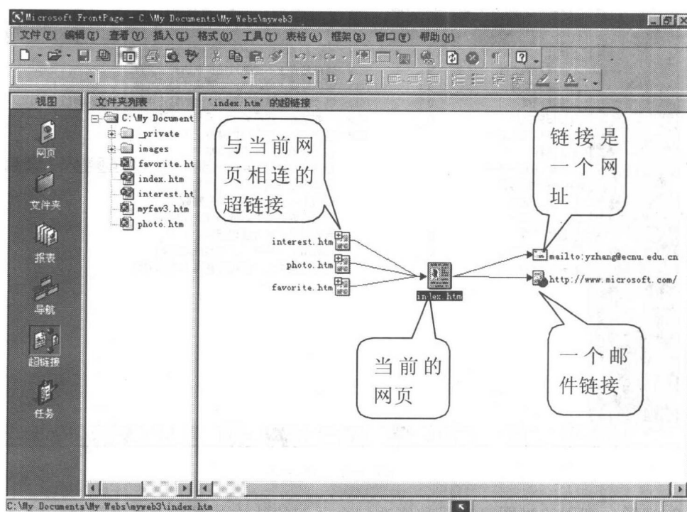
图 1-5 超链接视图
