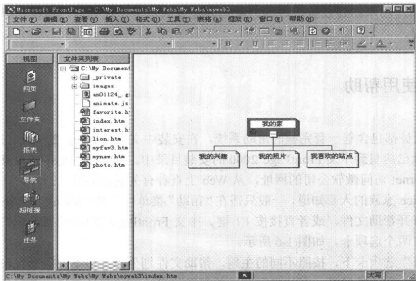
图 1-4 导航视图
