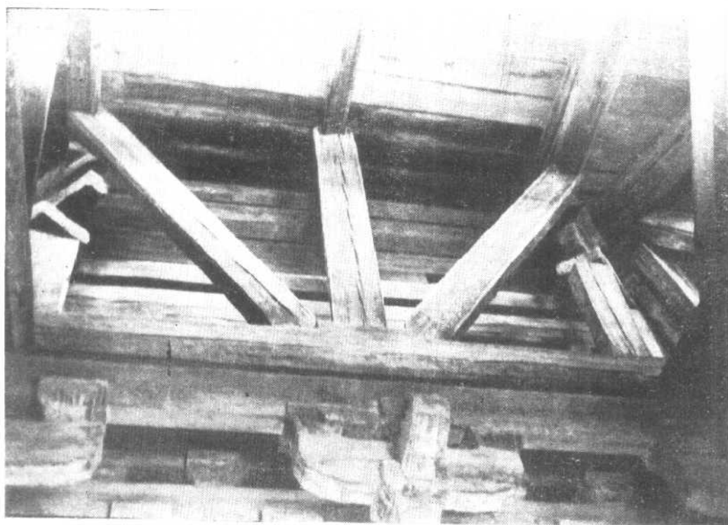
金代维修应县木塔时，在暗层中所加斜撑
