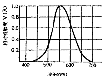
图 1.1.7 相对视敏函数曲线
