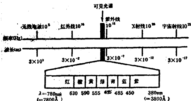
图 1.1.1 电磁辐射波谱
