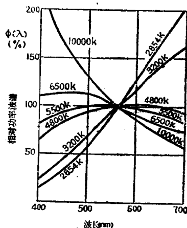
图 1.1.6 各种色温的黑体辐射的光谱分布
