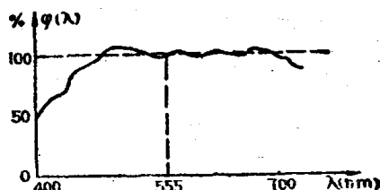
图 1.1.2 太阳辐射的相对功率波谱
