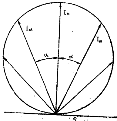
图 1.1.8 漫散射面光源的发光强度分布
