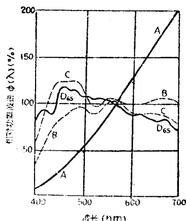
图 1.1.5 标准光源的光谱分布
