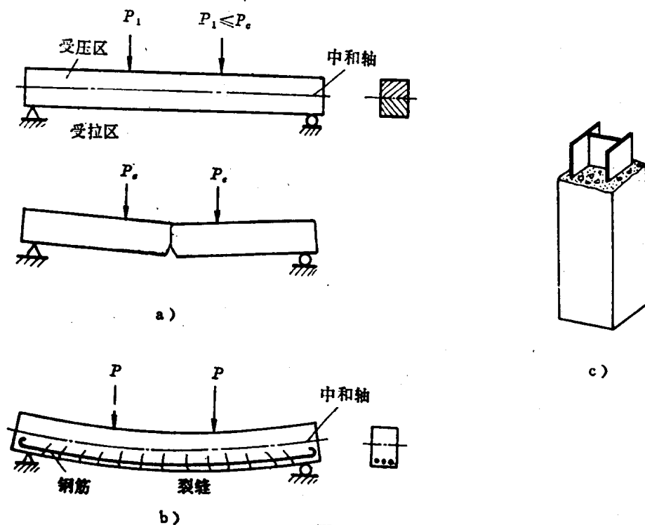
图0-1 钢筋混凝土
