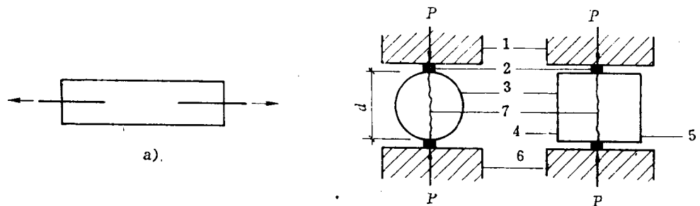
用圆柱进行劈裂试验 用立方体进行劈裂试验 b)
