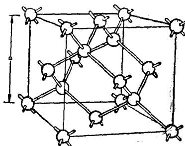
图 2.1(a) 闪锌矿结构
