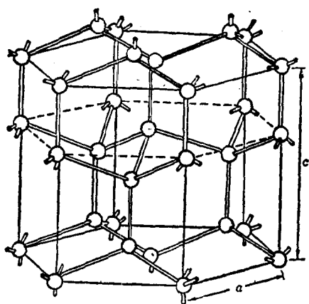
图 2.1(b) 纤锌矿结构
