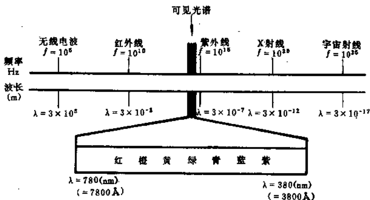
图 1-1 电磁辐射波谱
