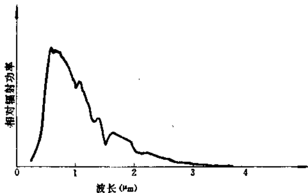
图 1-2 太阳辐射功率波谱
