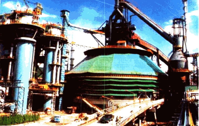
首钢二号高炉1991年采用新技术大修改造后全貌
