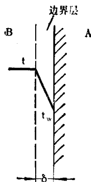
图 2-2 沿平壁流动的对流传热
