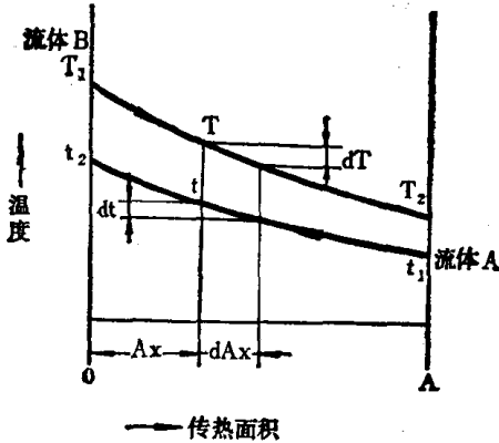
图 3-2 逆流热交换器中的温度分布
