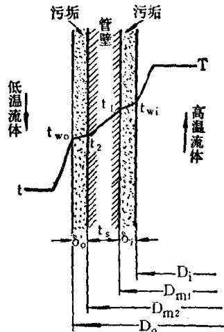
图 2-3 热交换器中的传热
