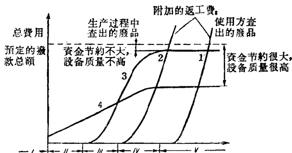
图 1 各不同設計阶段的費用分布
