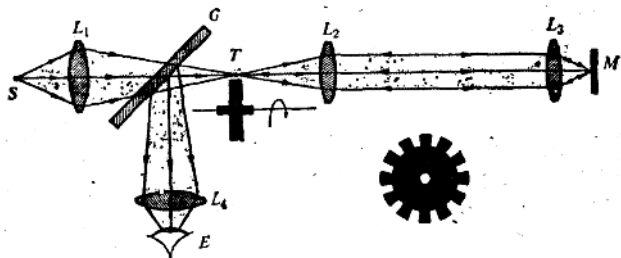
图38-5 斐索测量光速的齿轮法。 S 为光源， L_1 、 L_2 、 L_3 和 L_4 为透镜。 T 为齿轮， M 为反射镜， G 为玻璃板。
