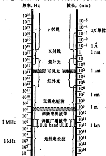
图 38-3 电磁波谱图
