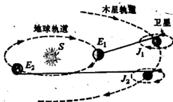
图38-4. 罗末推算光速的方法。
