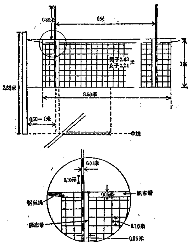
图3 球网设备、设置
