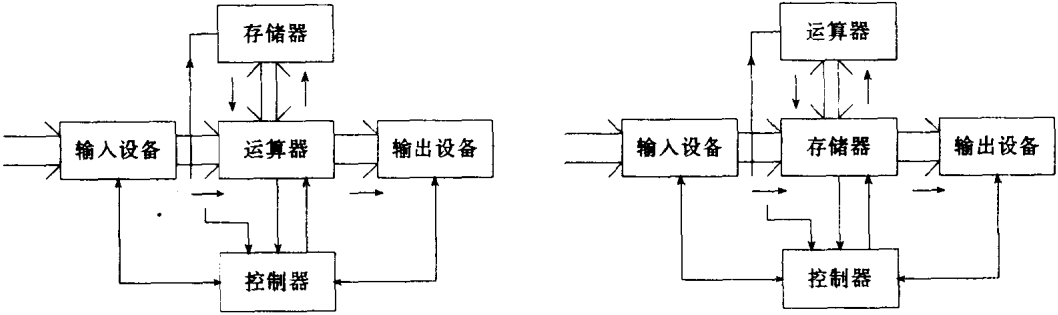
(a) 以运算器为中心的计算机 (b) 以存储器为中心的计算机
