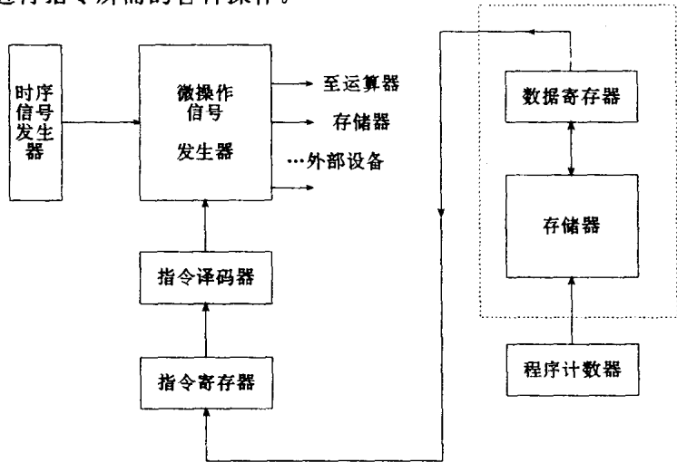
图 1-2 控制器原理框图
