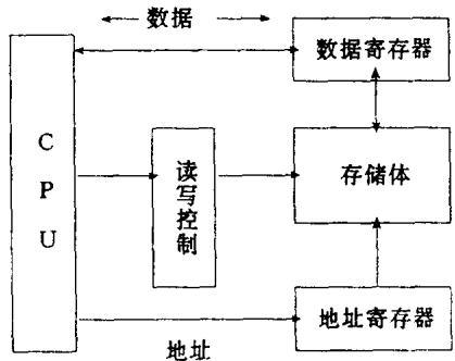
图 1-3 存储器原理框图
