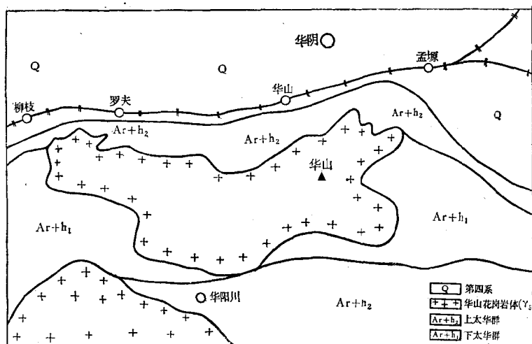
图 2 华山地质略图
