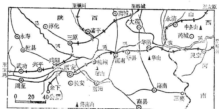
图 1 华山交通位置图
