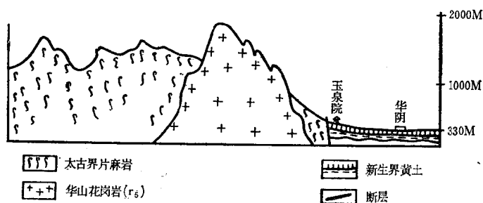
图 5 华山山麓地质剖面示意图
