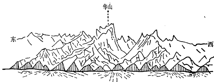
图 6 华山的断层三角面与断层崖
