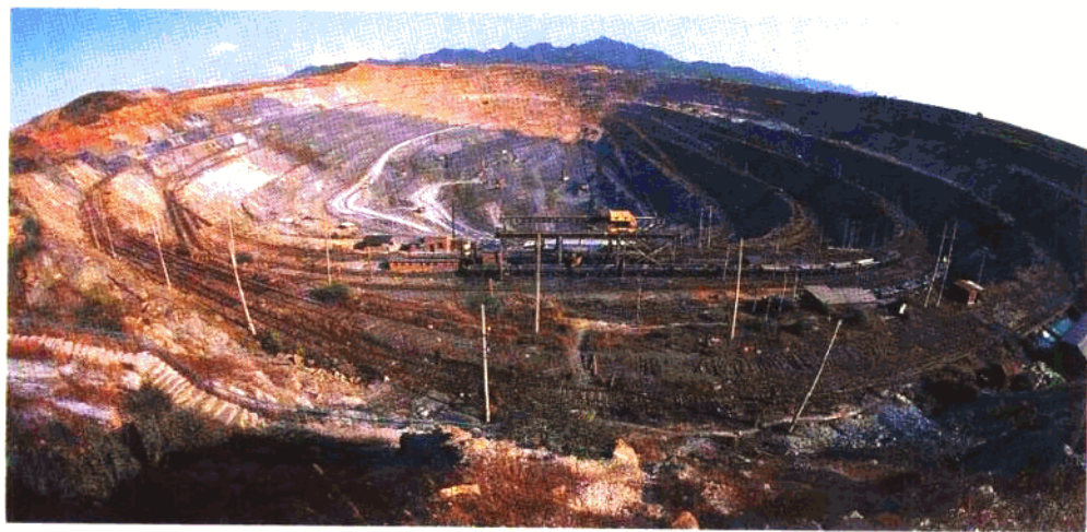
· 鞍钢矿山公司大孤山铁矿采场
