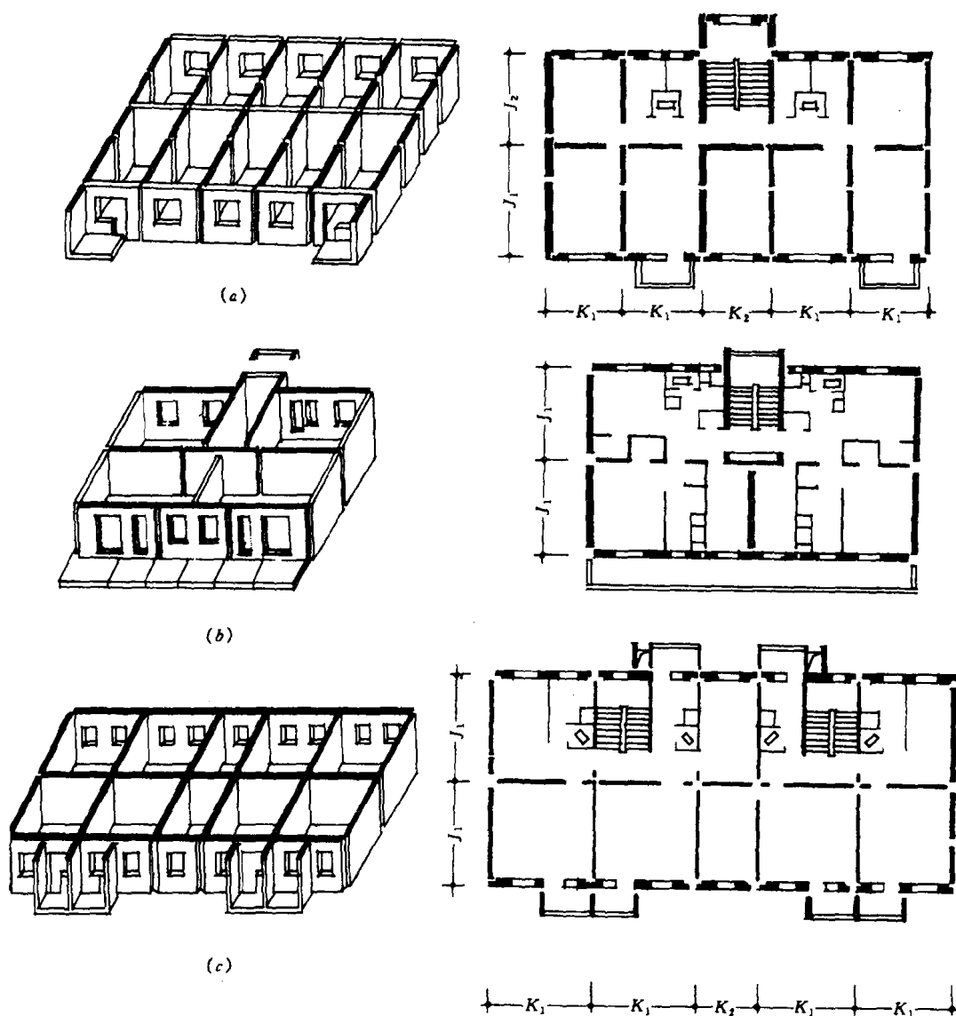
图 1-6 大板建筑承重方案
