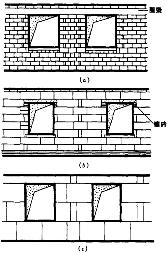
图 1-2 砌块排列示意
