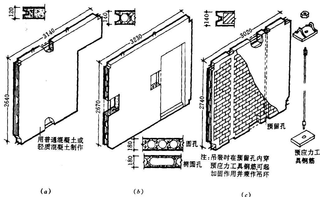
图 1-8 各种内墙板
