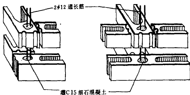
图 1-4 空心混凝土砌块建筑的芯柱
