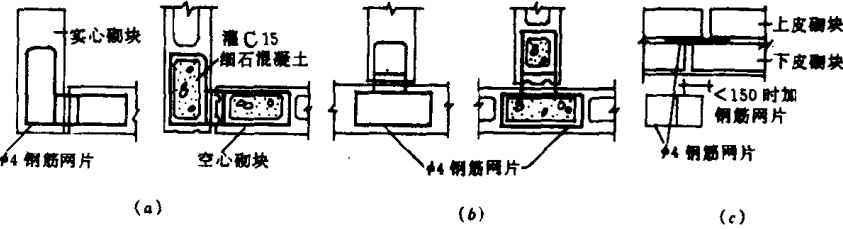
图 1-3 通缝处理
