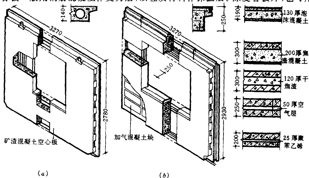
图 1-9 各种外墙板
