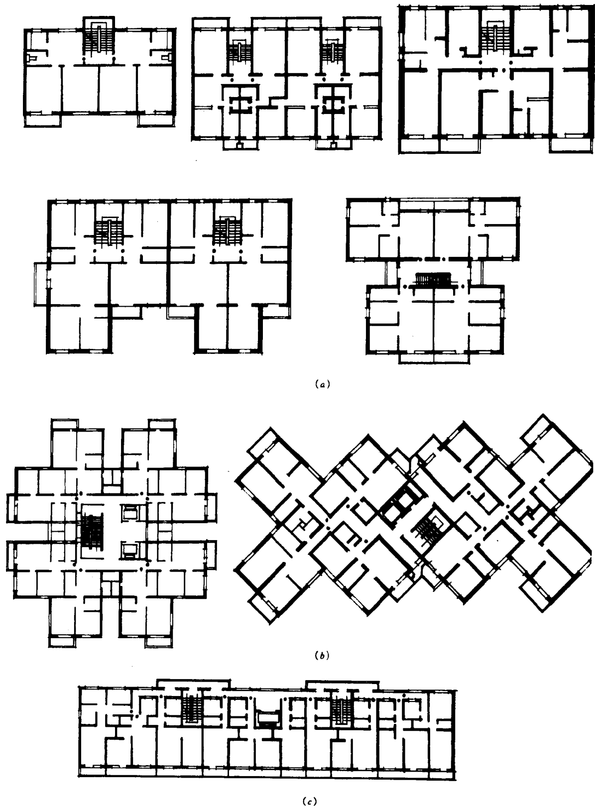
图 1-7 大板住宅平面示例
