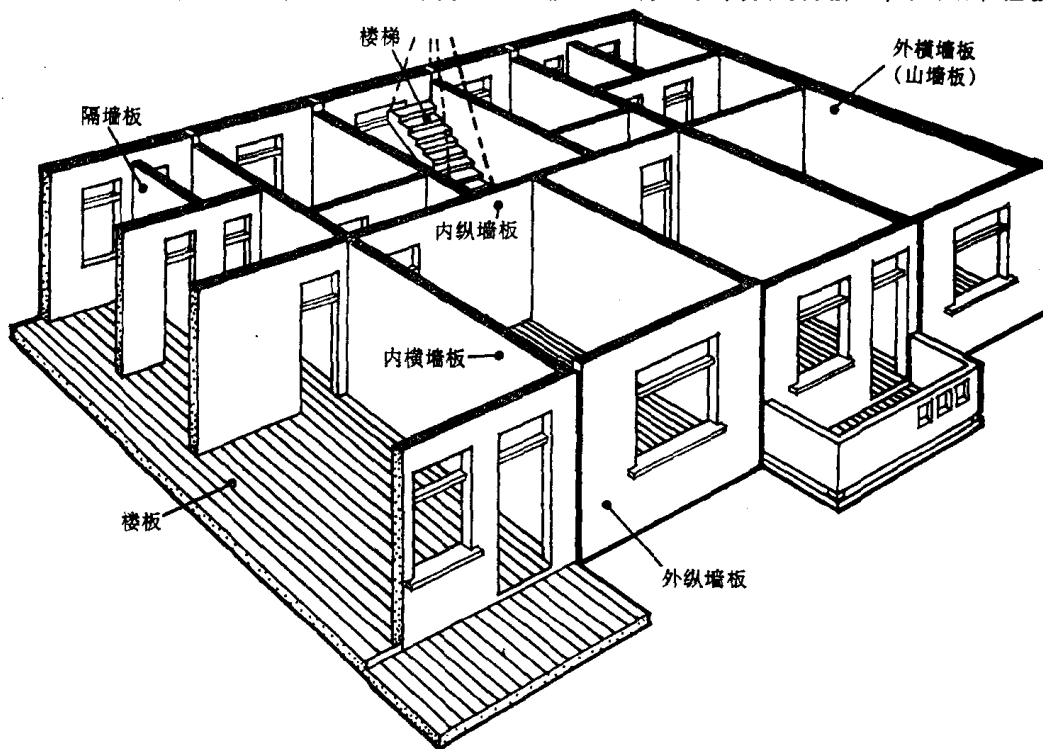
图 1-5 大板建筑
