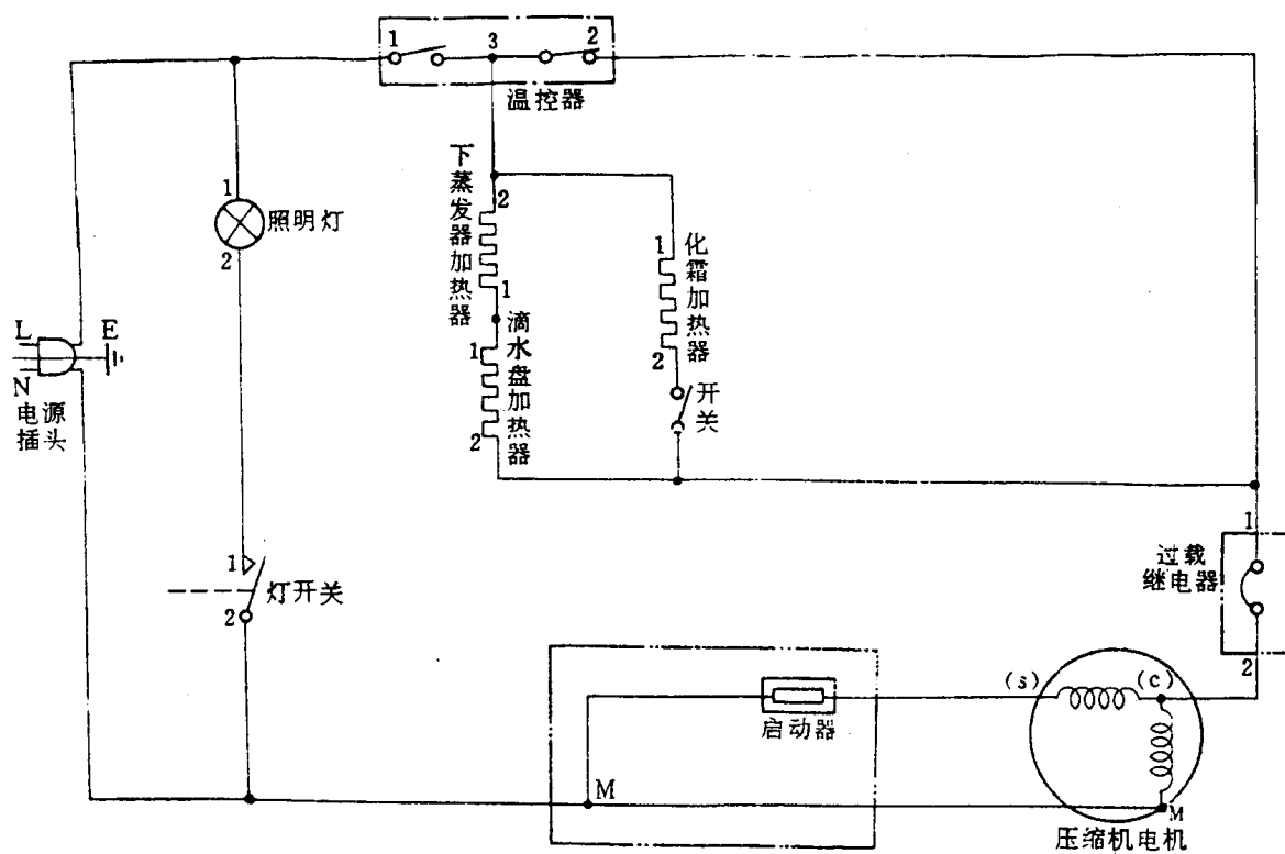
图 1-1 航天牌 BCD-140 电冰箱电气原理图
