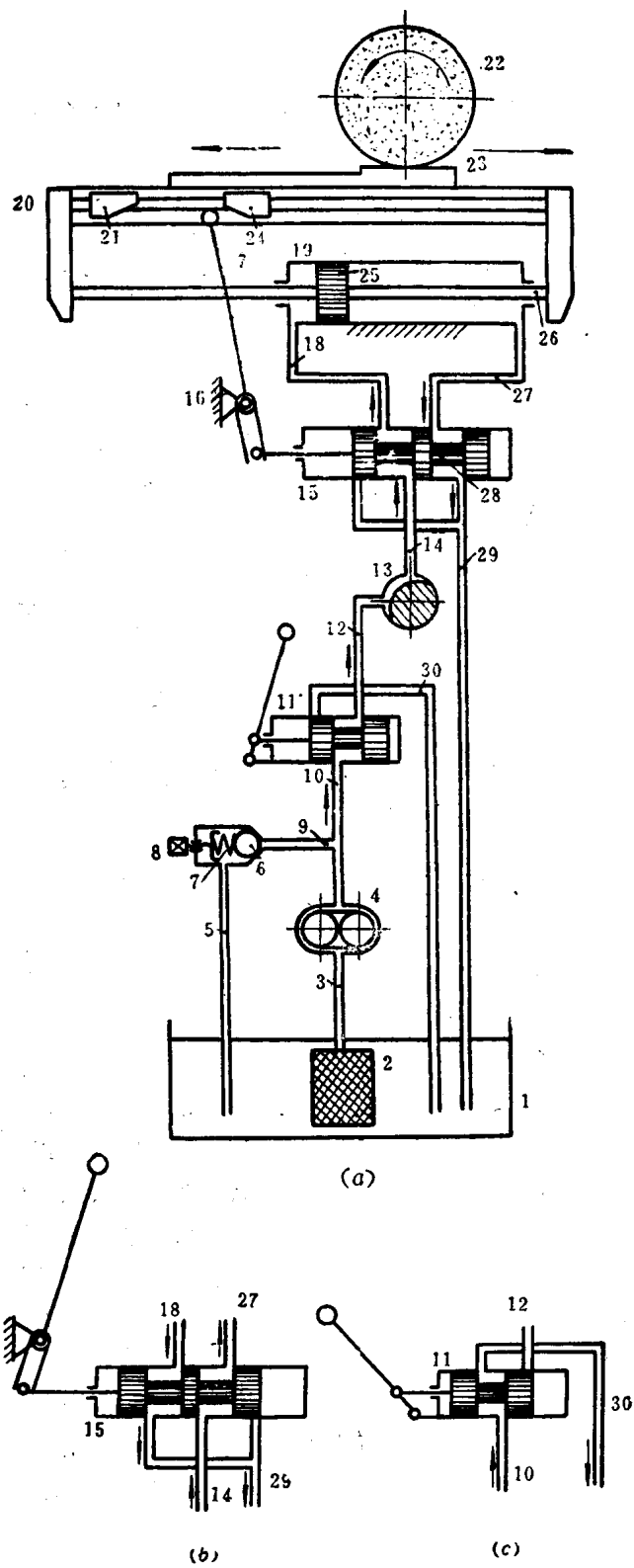
图 1-1 磨床工作台液压系统工作原理图 (半结构图)
