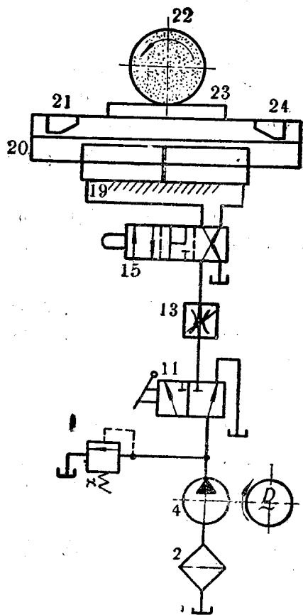
图1-2 磨床工作台液压系统工作原理图（职能符号图）
