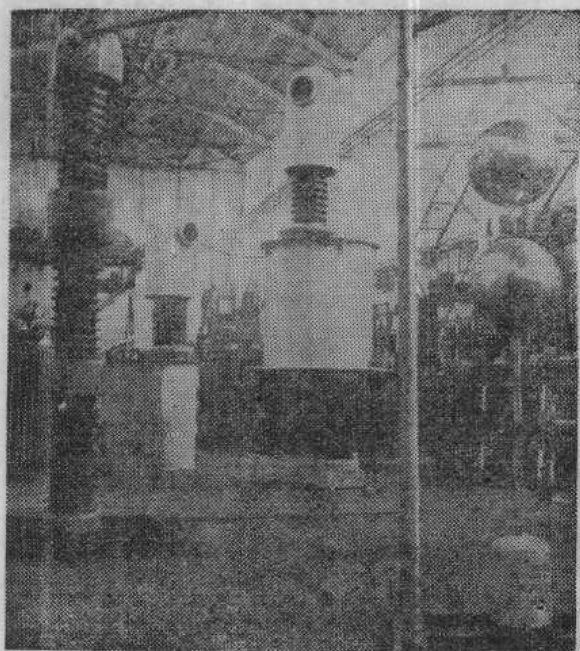
图 1—5 500 千伏安 500 千伏 试验变压器、水 阻器和球隙器
