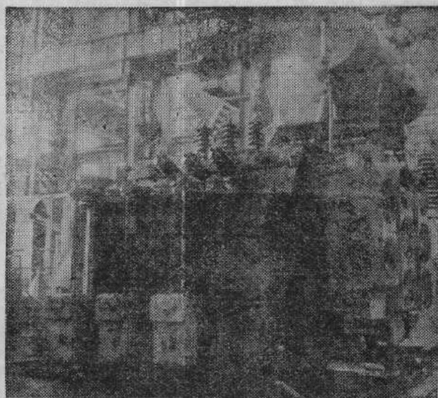
图1—4 (a) ZSFPT— 40000/35 整流变压 器
