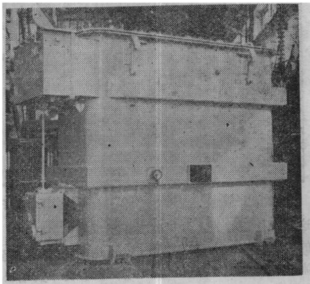
图 1—3 (a) HSPF—10000/10 矿热炉变压器
