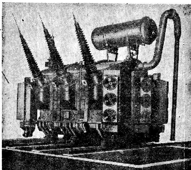
图 1—1 SFP—120000/220 120000 千伏安，220 千伏升压变压器
