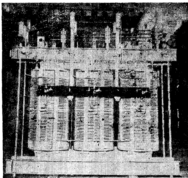
图 1—2 (b) SG—750 千伏安干式变压器器身
