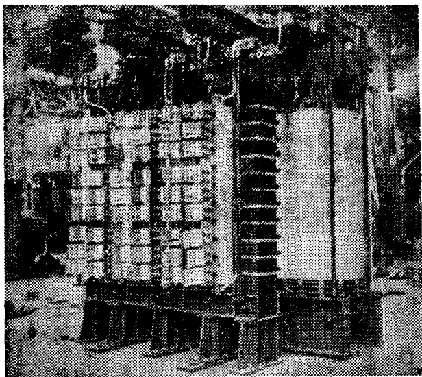
图 1—3 (b) HSSPZ—18000/35 电炉变压器器身
