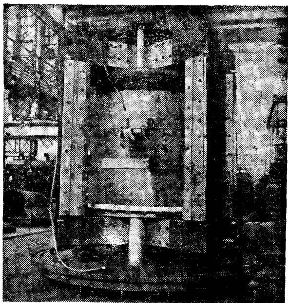
图1—7 (b) BKDFP—30000/330 并联电抗器器身
