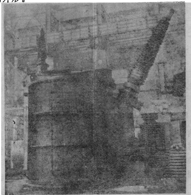
图1—7 (a) BKDFP—30000/330 并联电抗器
