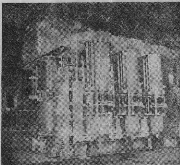
图1—4 (b) ZSFPT— 40000/35 整流变压 器器身
