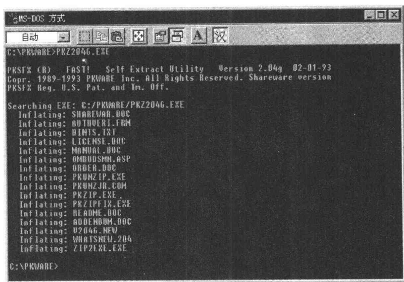
图 3-1 执行 PKZ204G.EXE 的画面
