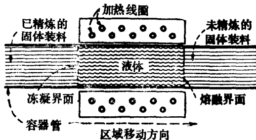
图 17-5 区域熔炼简图
