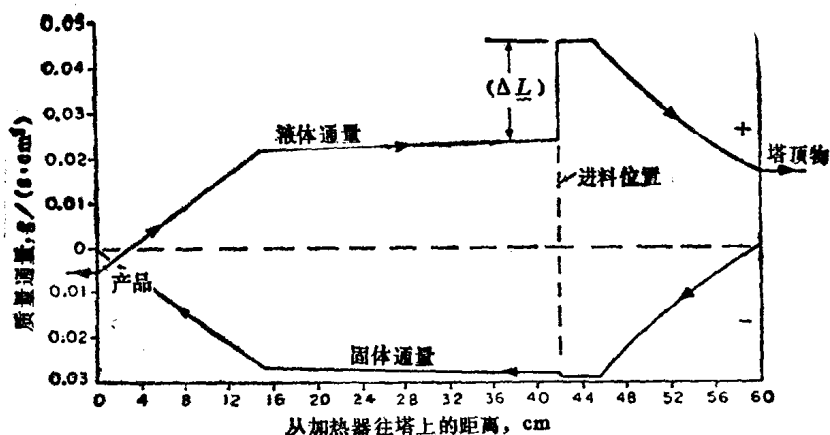
图 17-13 紧密床层塔式结晶器中计算出来的液体和固体通量
