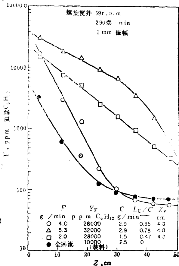
图 17-10 全回流下偶氮苯和茈在中央加料塔式结晶器中的稳态分离 (Zief and Wilcox, Fracton: Solidification , vol 1, Marcel Dekker, New York, 1967, p. 356)
