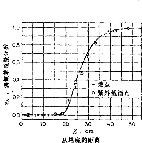
图 17-10 全回流下偶氮苯和茈在中央加料塔式结晶器中的稳态分离 (Zief and Wilcox, Fracton: Solidification , vol 1, Marcel Dekker, New York, 1967, p. 356)
