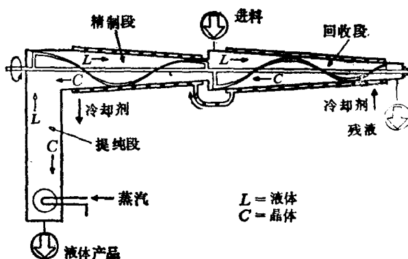
图 17-8 横卧式中央加料塔式结晶器
