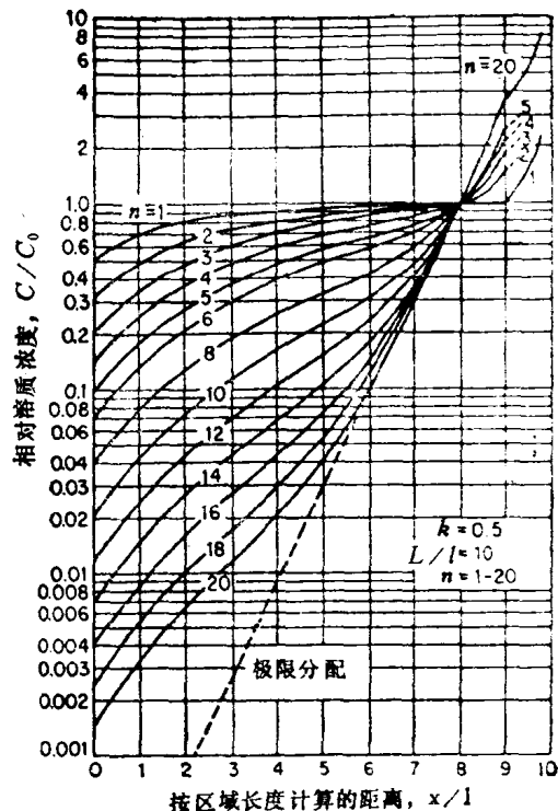
图 17-6 对不同程数 n , 相对溶质浓度 C/C_0 (对数坐标) 对区域长度距离 x/l (从装料开始处算) 的标绘 (Pfann, Zone Melting , 2d ed., Wiley, New York, 1966, p. 290.)
