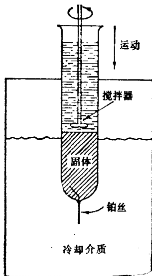
图 17-3 正常冻凝设备
