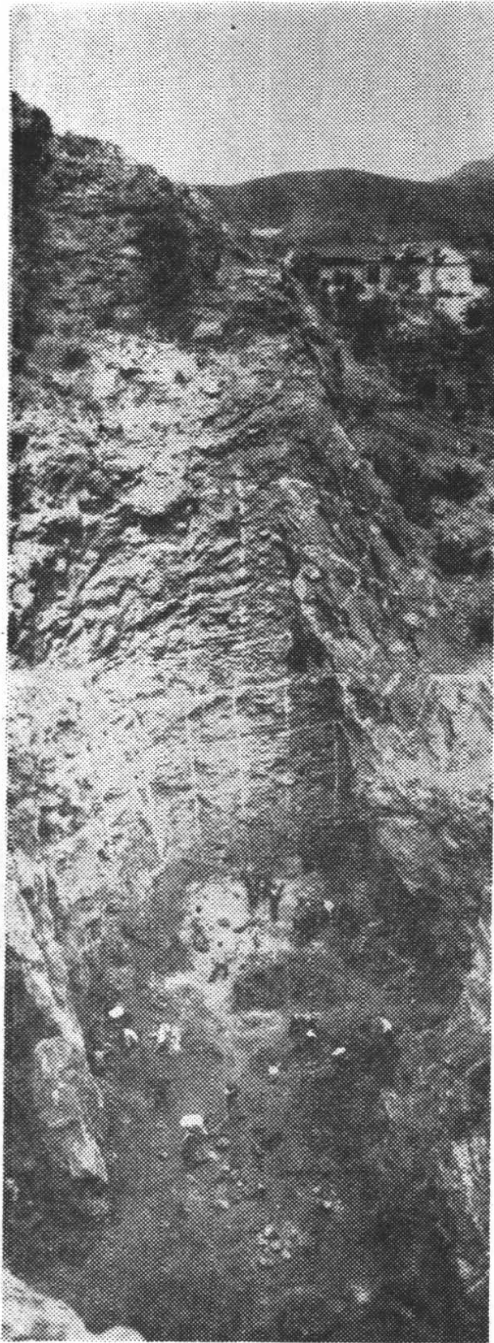
中国猿人遗址的底部(第 13 层) 发掘情形。
