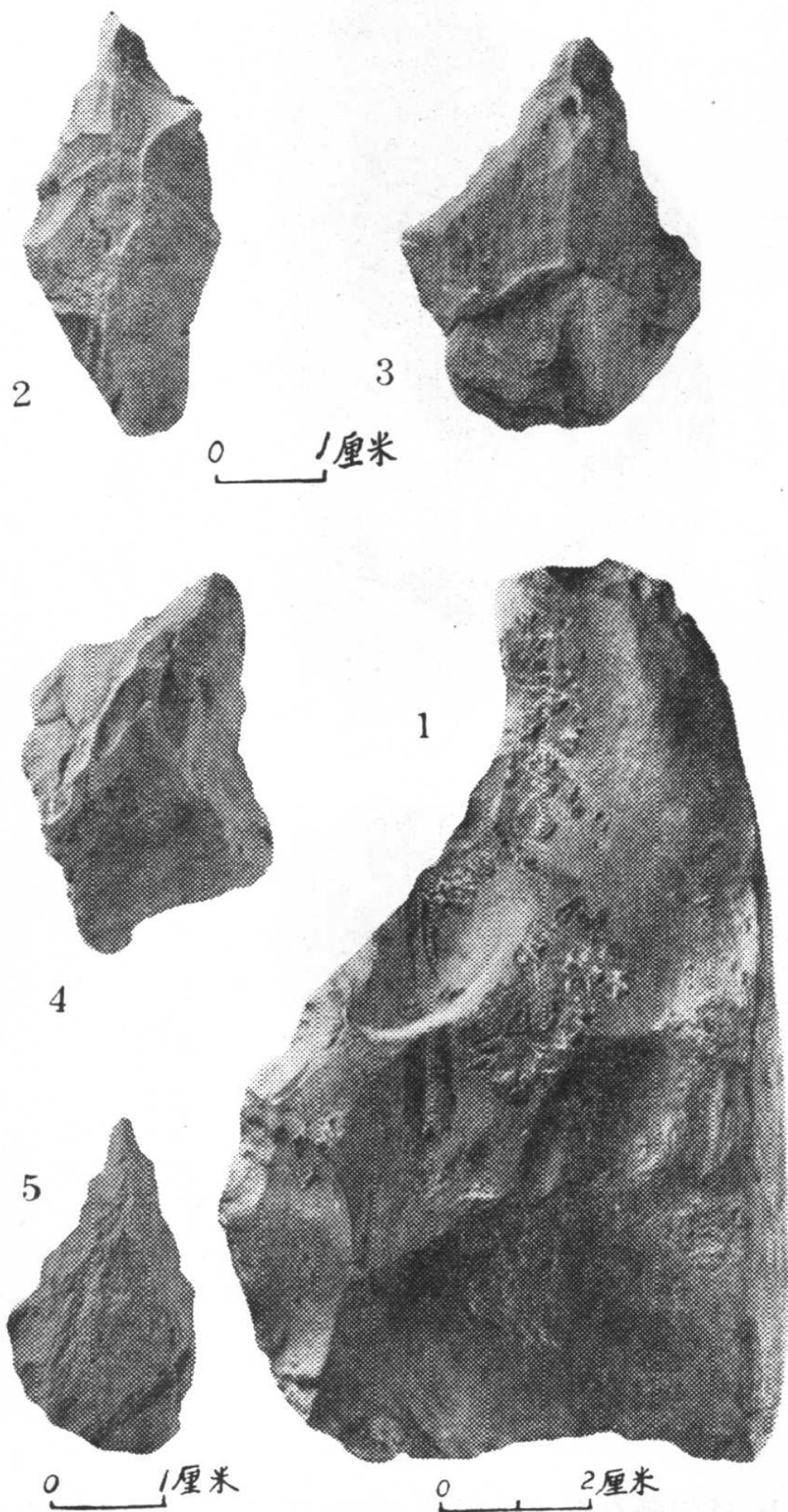
1,两面加工的燧石砍斫器;2,燧石尖状器;3及5,脉石英尖状器;4,脉石英斜尖尖状器。
