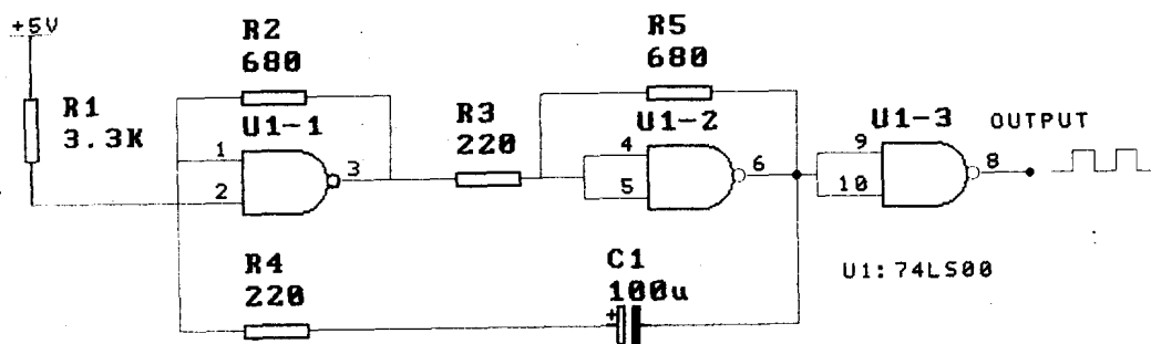
图 2.1(b) 信号源原理图
