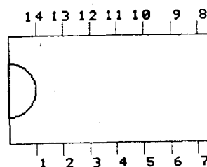
图 1.1 芯片引脚编号方式
