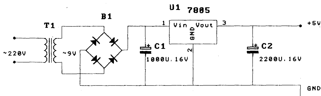
图 2.1(a) 稳压电源原理图
