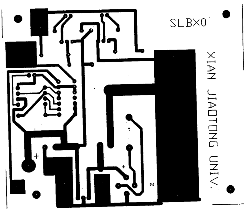
图 2.2 SLBX0 模块印刷电路板图
