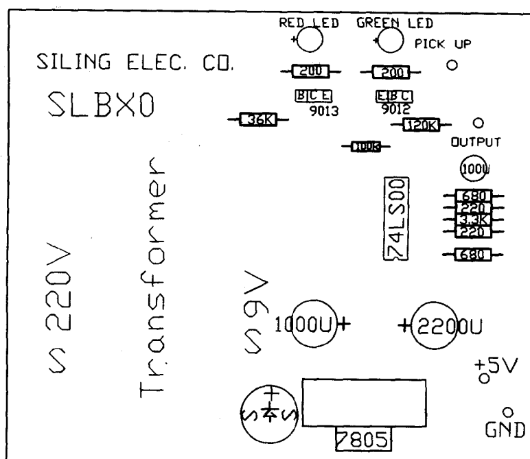
图 2.3 SLBX0 模块元件布置图
