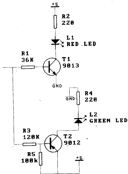
图 2.1(c) 逻辑测试器原理图
