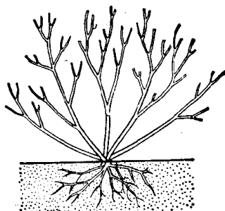
斜升茎
