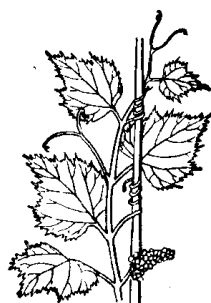
攀援藤本
