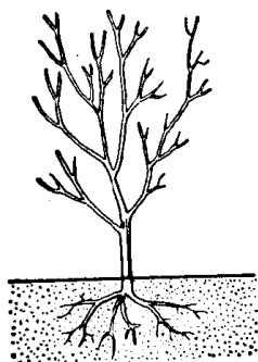
直立茎
